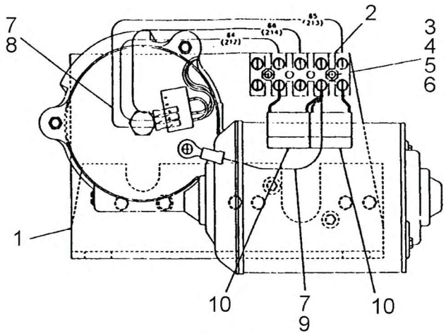
VIEW A-A
